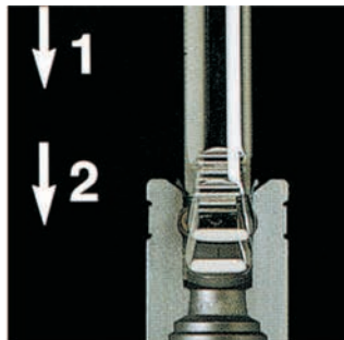
Dwa stopnie mocowania trzpienia Pierwszy pozwala na ruch w bok do 30 stopni, drugi blokuje przedłużkę w pionie na stałe
