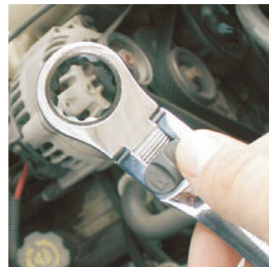
Jednopalcowy przełącznik blokady położenia grzechotki
